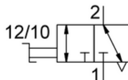
3/2 vias
