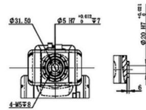
Diagrama de instalação da flange
